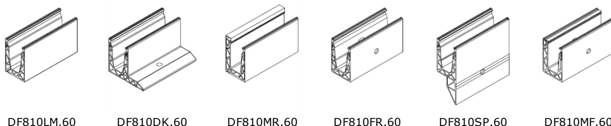
Figure 2 - Profils de support de la gamme DEFENDER 810
